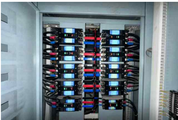
전력인입점 분전함(내부)
