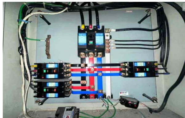
전력인입점 분전함(내부/L3B)
