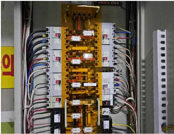
지하주차장 분전함(P-P31 PANEL)-내부
